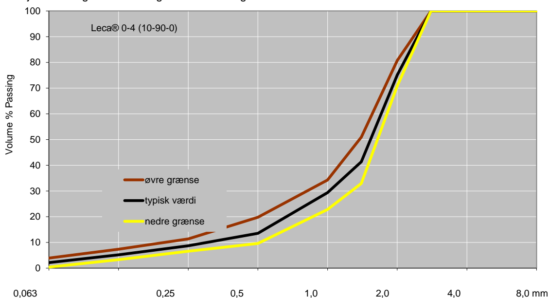
Vejledende sigtekurve omregnet til volumen gennemfald
