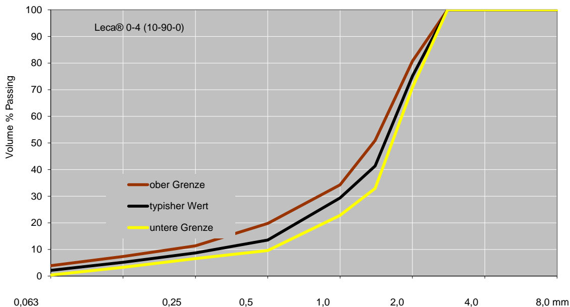
Richtungsweisende Siebkurve in Volumen-Durchgang umgerechnet
